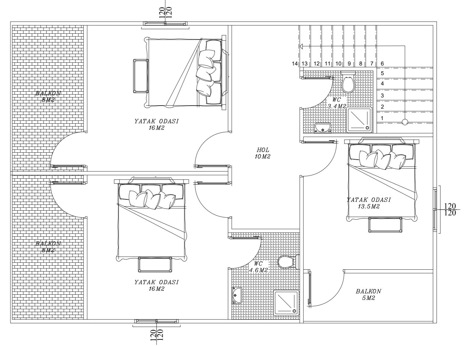
BİRİNCİ KAT PLANI ALAN: 101 M2
