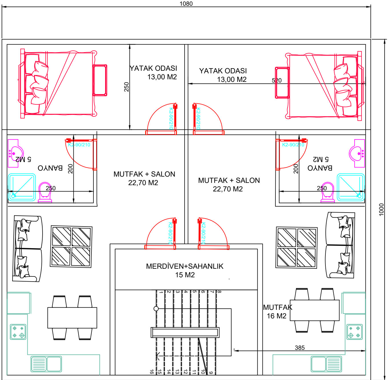
AYVALIK HACİVELİLER 108+108 DIŞTAN MERDİVENLİ 1.KAT
